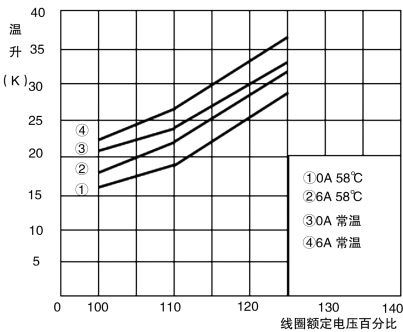
线圈温升
