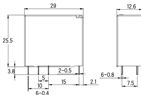
外形尺寸图
